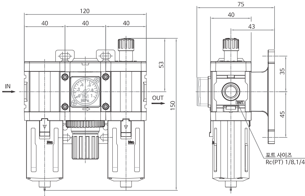
MAU 201 (콤비네이션형, 필터+레귤레이터+루브리케이터)
