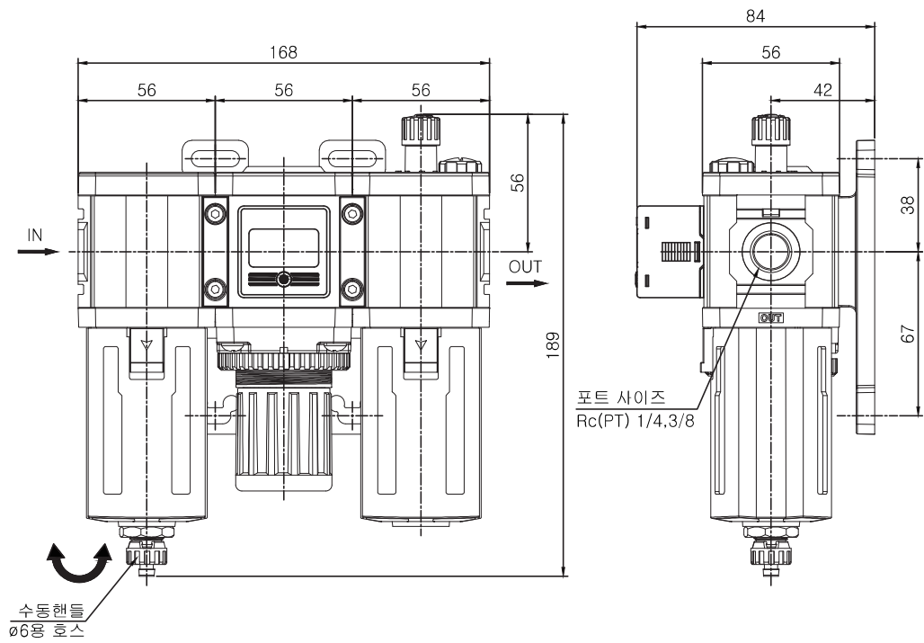
MAU301 (콤비네이션형, 필터+레귤레이터+루브리케이터)
